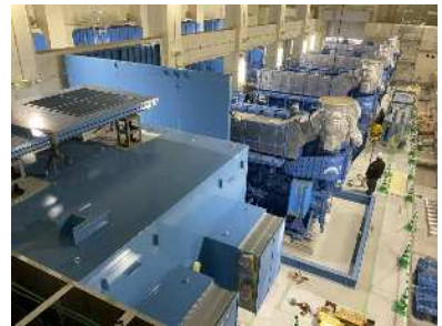
原動機パッケージ組立状況
