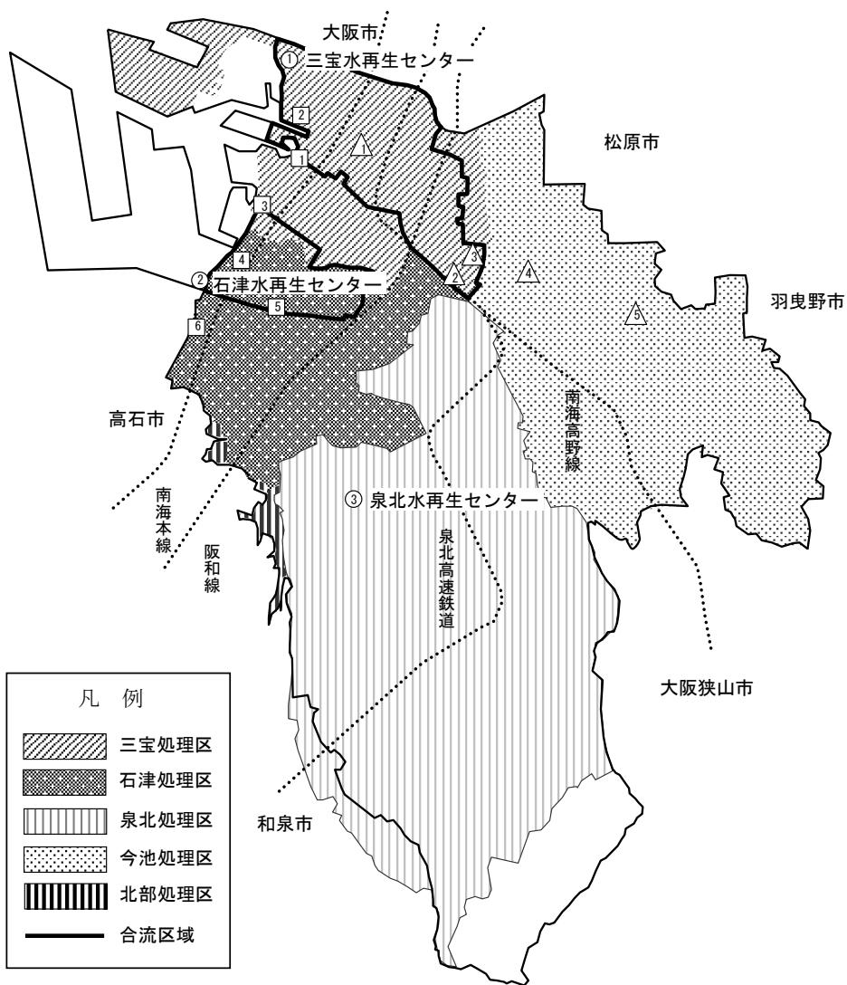
○下水道施設位置と全体計画区域図
