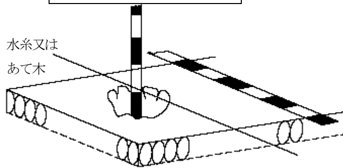
砕石基礎工（転圧完了後）
