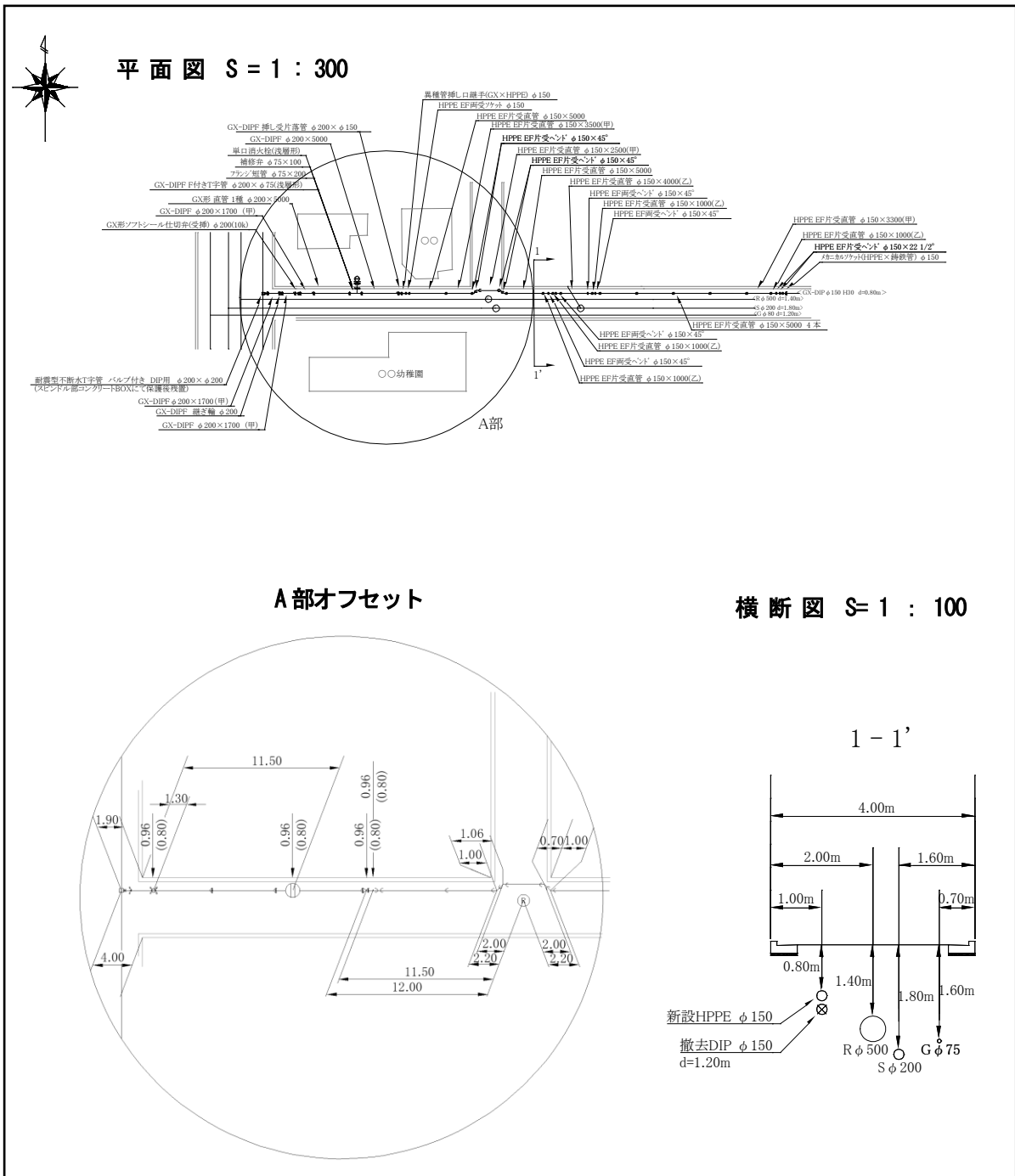
図2-8 平面図・横断図作図例
