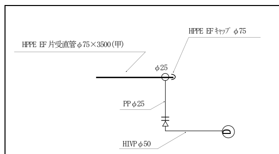
図2-9 排水栓（呼び径25mm）作図例
