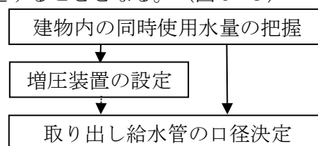
図9-5 増圧方式給水における口径決定の手順
