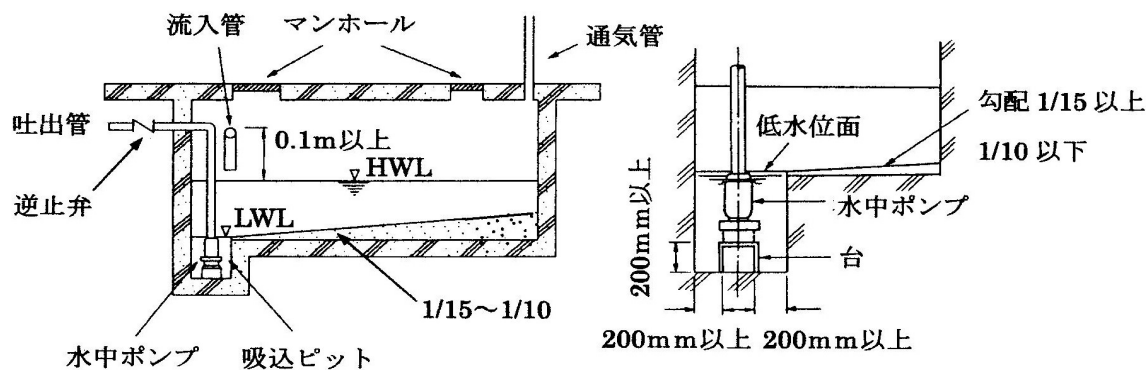
図 19 排水槽の例
