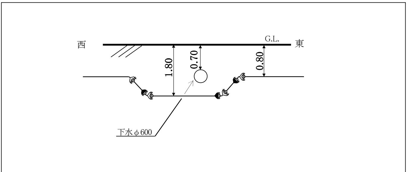
図5-6 伏せ越し図作図例
