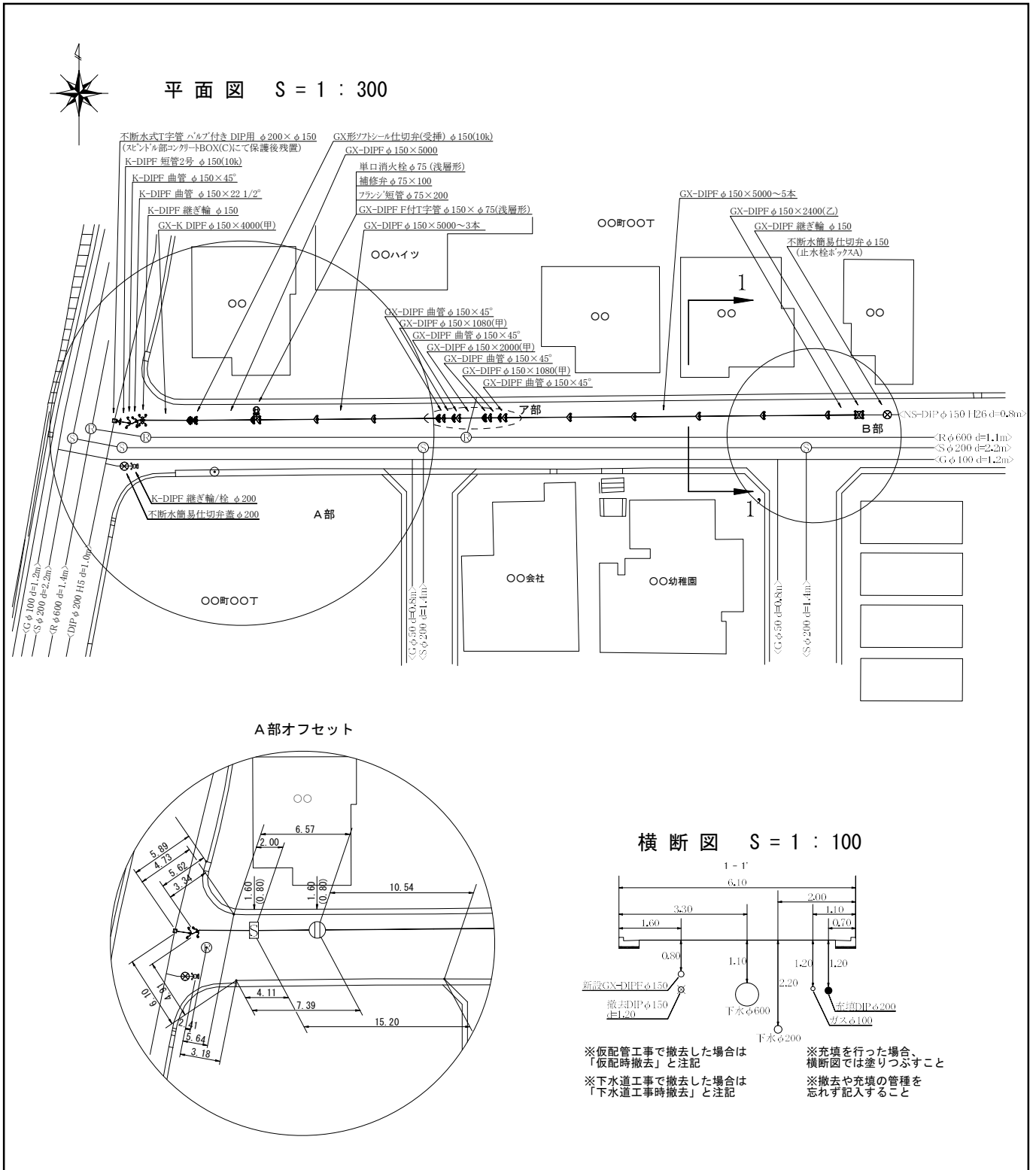
図5-3 平面図・横断図作図例
