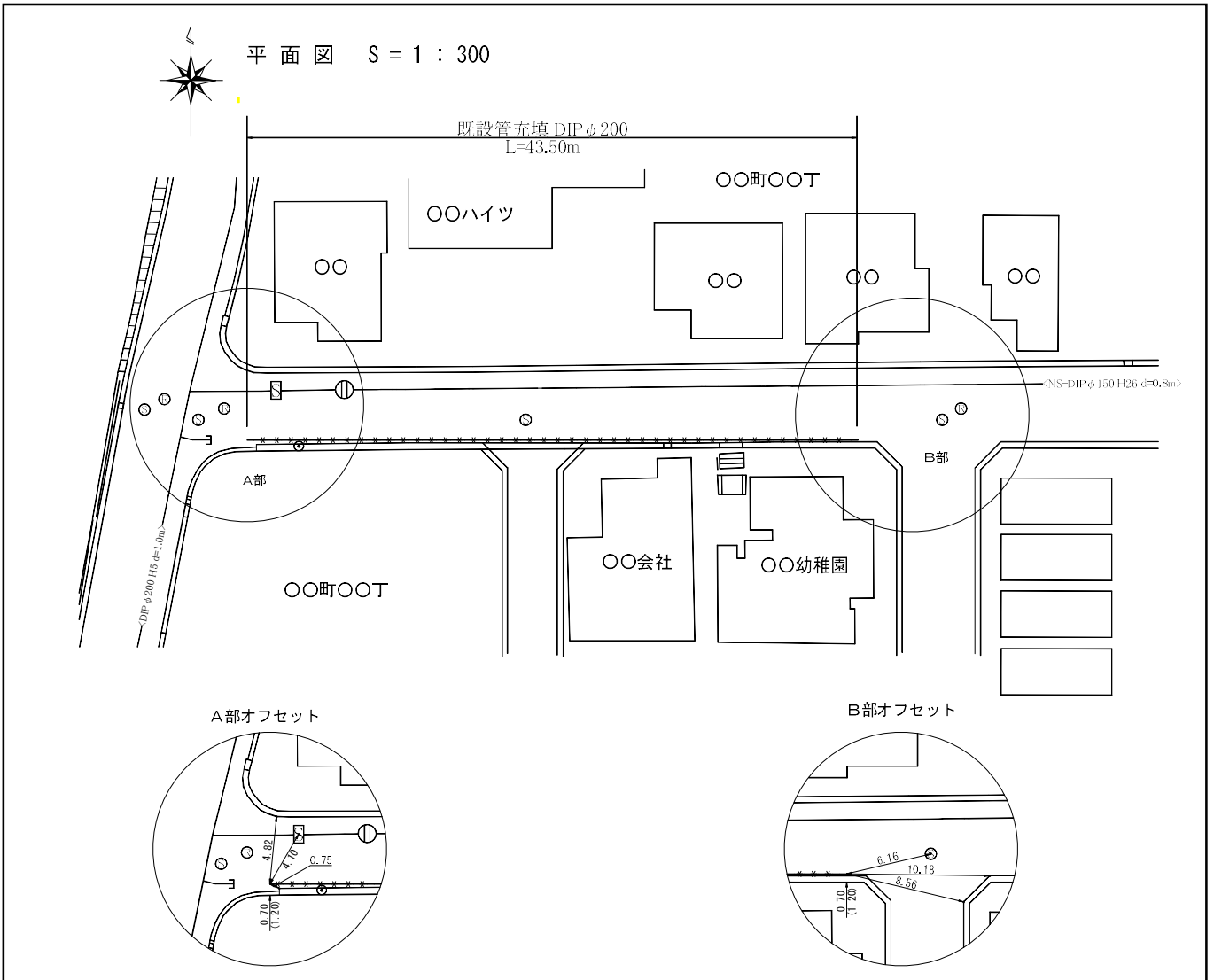
図5-5 オフセット起・終点参考図作図例2
