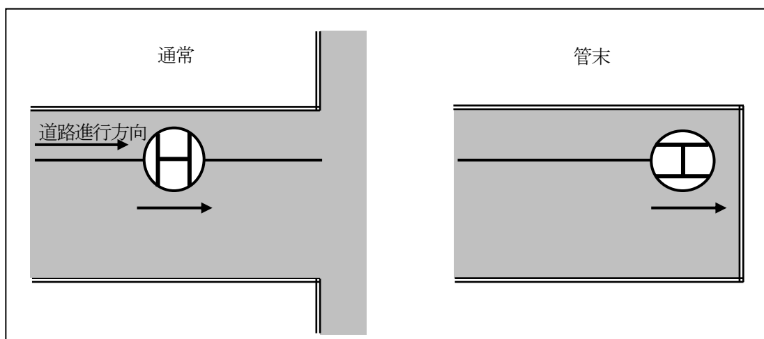
図2-4 消火栓及び空気弁の弁栓ボックスの設置方向
