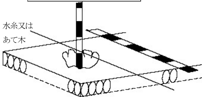
砕石基礎工（転圧完了後）
