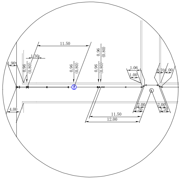
図5-3 平面図・横断図作図例
