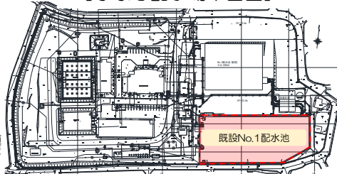
【家原寺配水場平面図】
