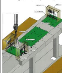
【ワイヤーソー工法概略図】
