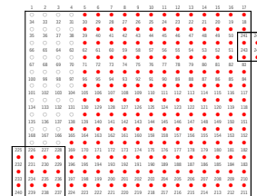
【基礎杭打設詳細図】
