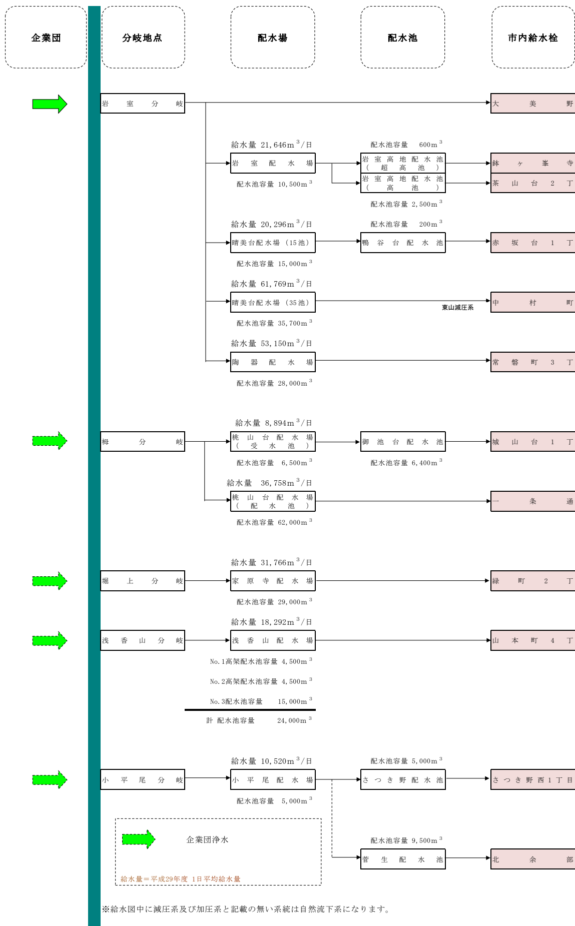
図2-1A 法令に基づく水質基準の検査に係る水質検査地点 (堺浜地区配水系統切替前)
