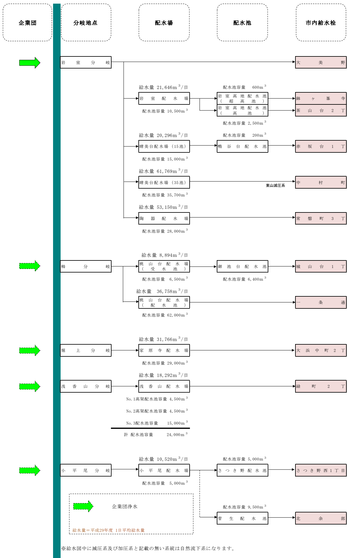
図2-1B 法令に基づく水質基準の検査に係る水質検査地点 (堺浜地区配水系統切替後)
