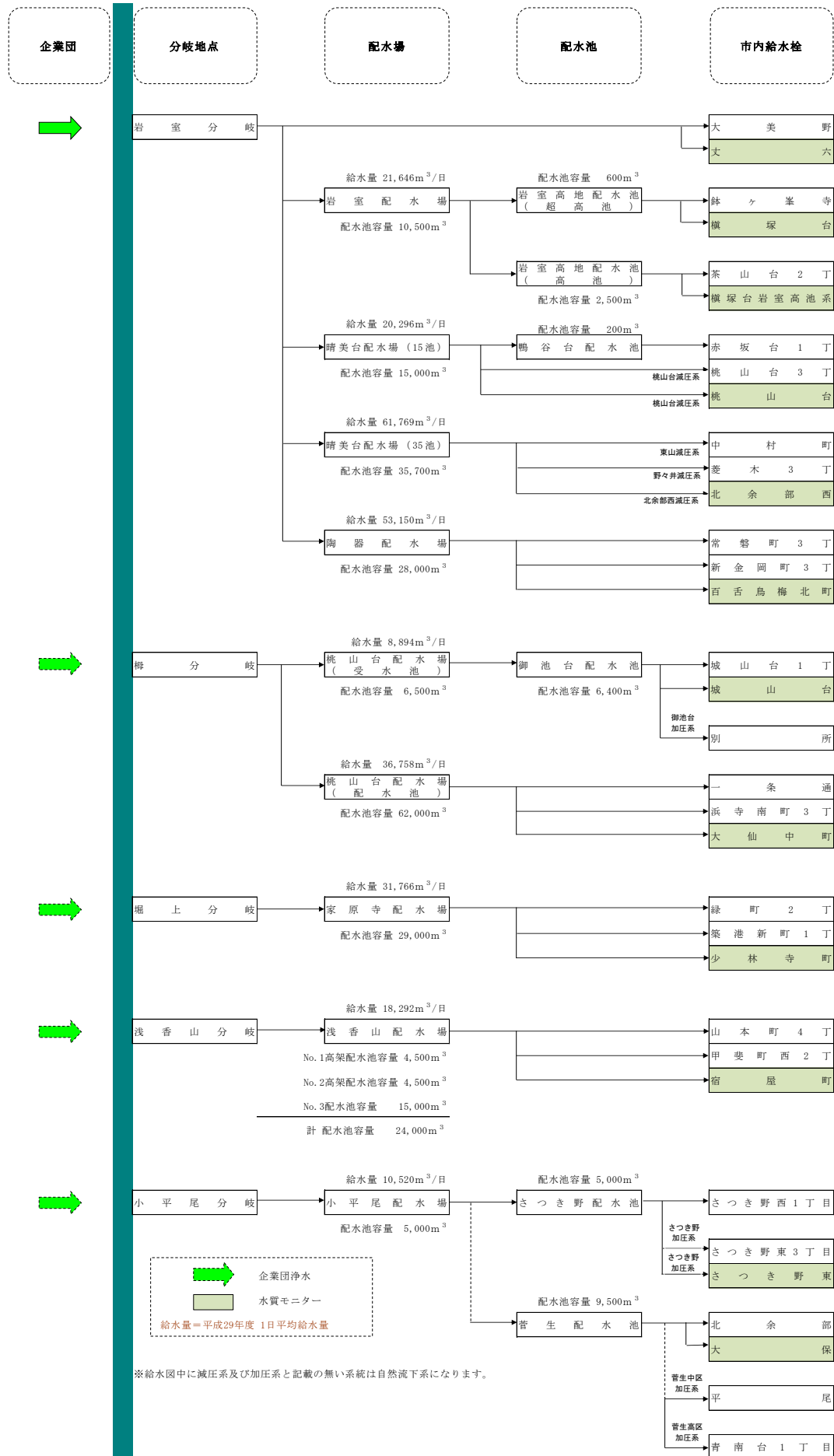
図2A 水質検査地点 (堺浜地区配水系統切替前)
