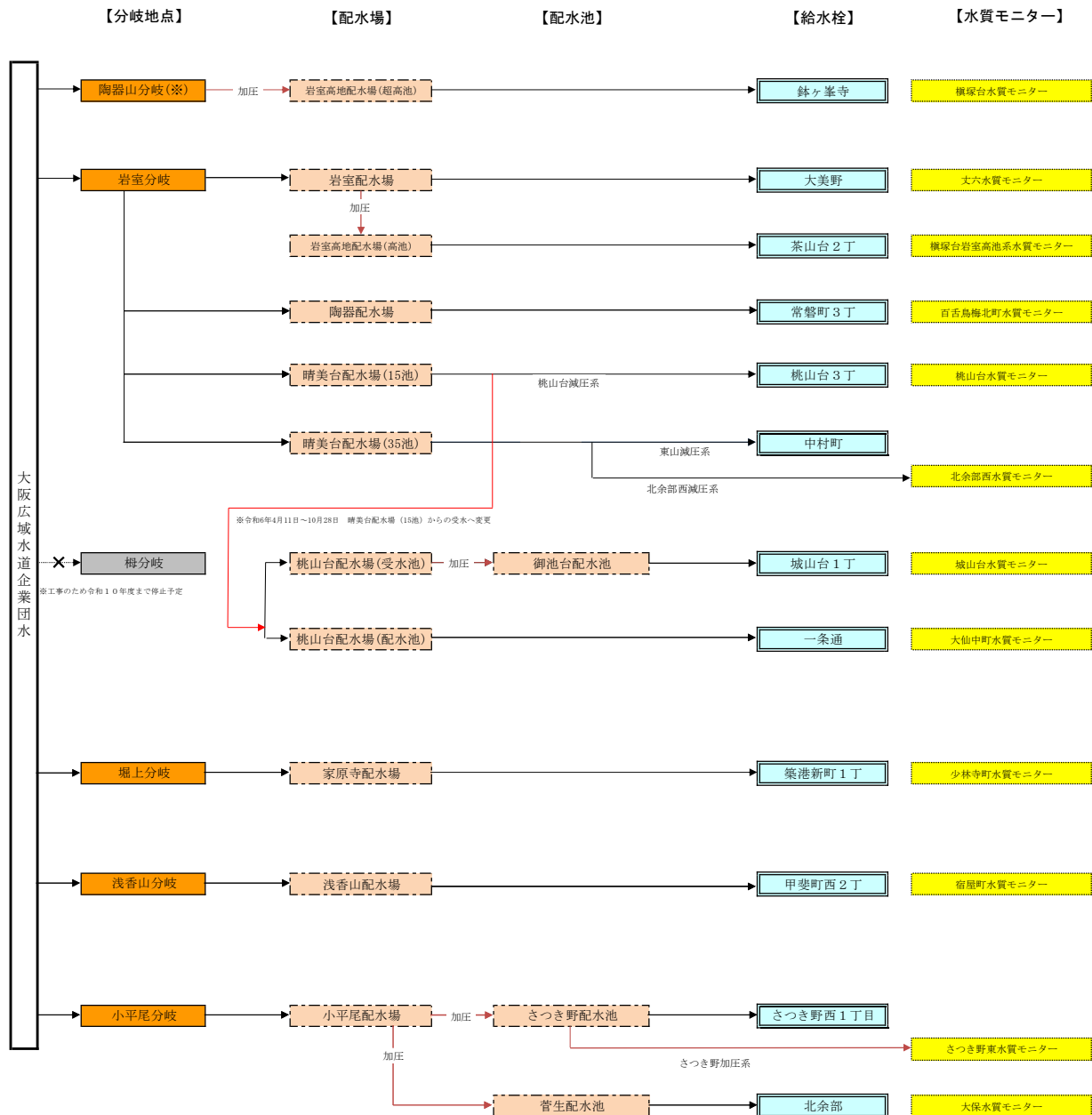
【 図 】 令和 6 年度水質検査地点（給水フロー図）（R6. 4. 11～10. 28）
