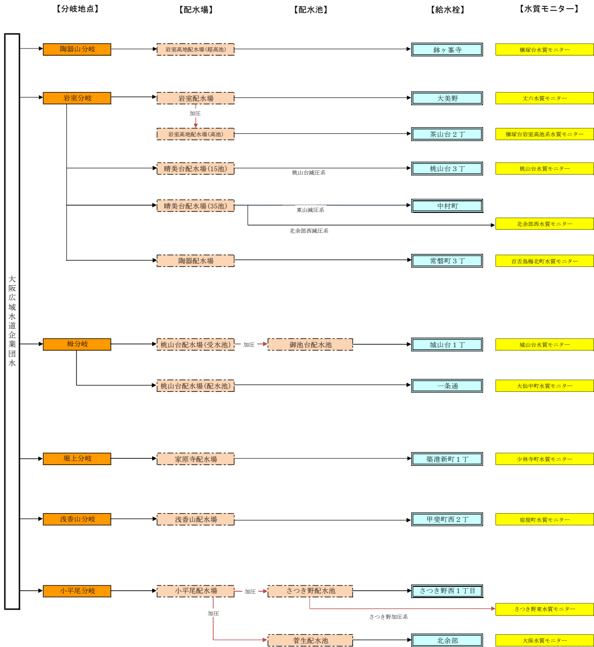
【 図 】 令和 6 年度水質検査地点（給水フロー図）（R6. 4. 1～4. 10）
